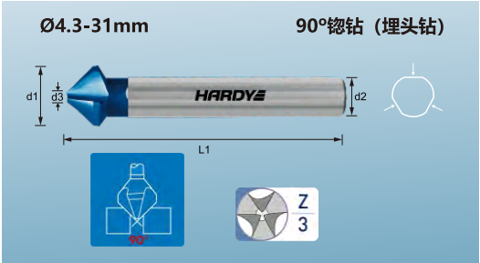
DIN335标准 C型 直柄 3齿 90°
