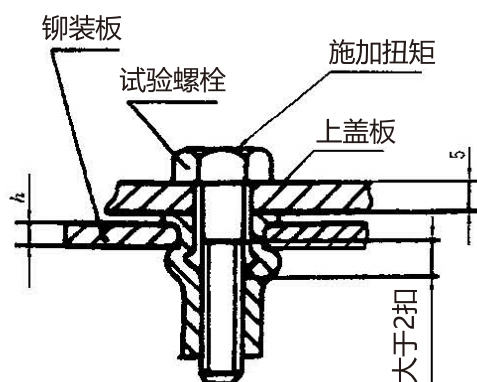
图4 破坏扭矩试验
