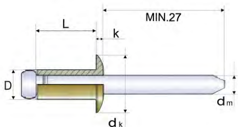
规格参数表 (尺寸单位: mm 强度单位: 牛顿)
