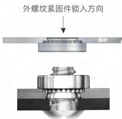
螺母压铆安装完成
