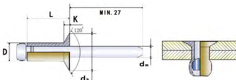
规格参数表 (尺寸单位: mm 强度单位: 牛顿)
