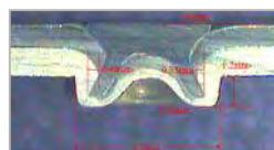
自冲铆参数示意图
