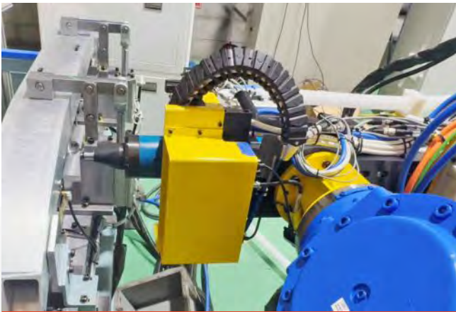
前保铆螺母自动铆接
