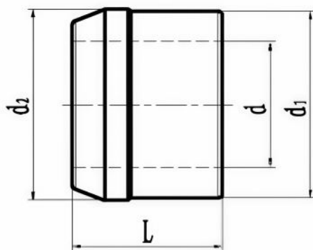
标准型套环
