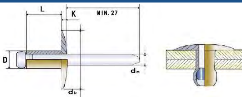
规格参数表 (尺寸单位: mm 强度单位: 牛顿)
